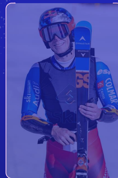
CLÉMENT NOËL
